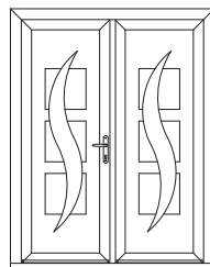
Nouvelle Zélande 2 vantaux.
