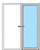
Porte-fenêtre, 1 vantail en galandage sur 1 rail
