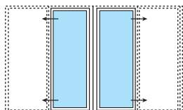
Porte-fenêtre, 2 vantaux en galandage sur 1 rail
